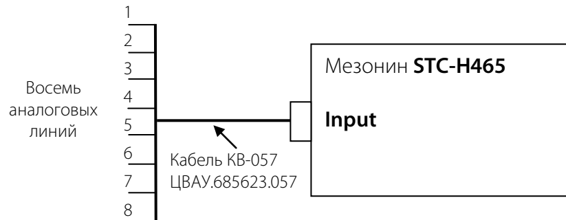
Рисунок 10 – Схема подключения мезонина STC-H465
