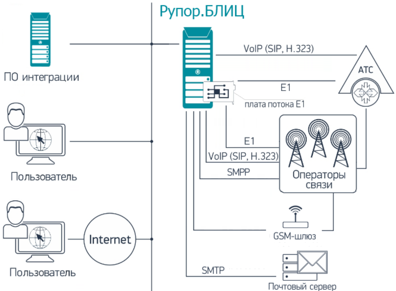
Рисунок 1 – Общая структура комплекса «Рупор.БЛИЦ»
