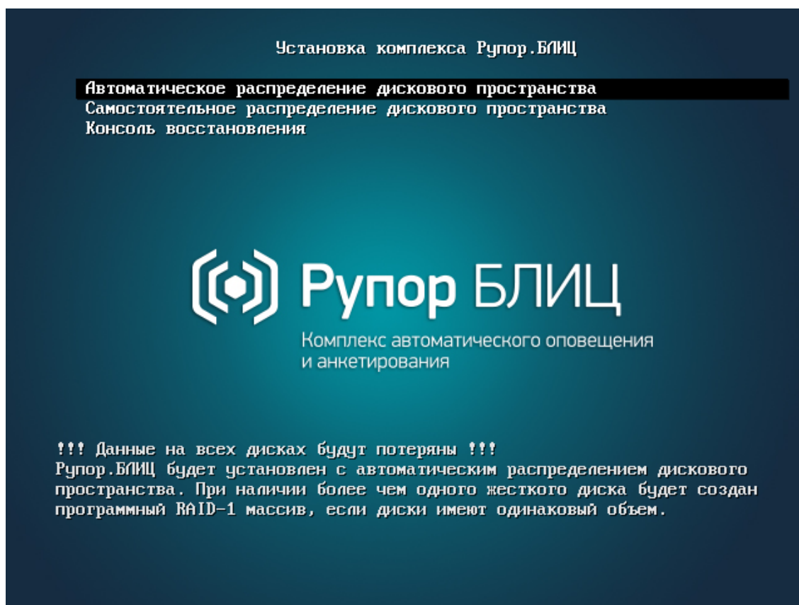
Рисунок 3 – Выбор типа установки
