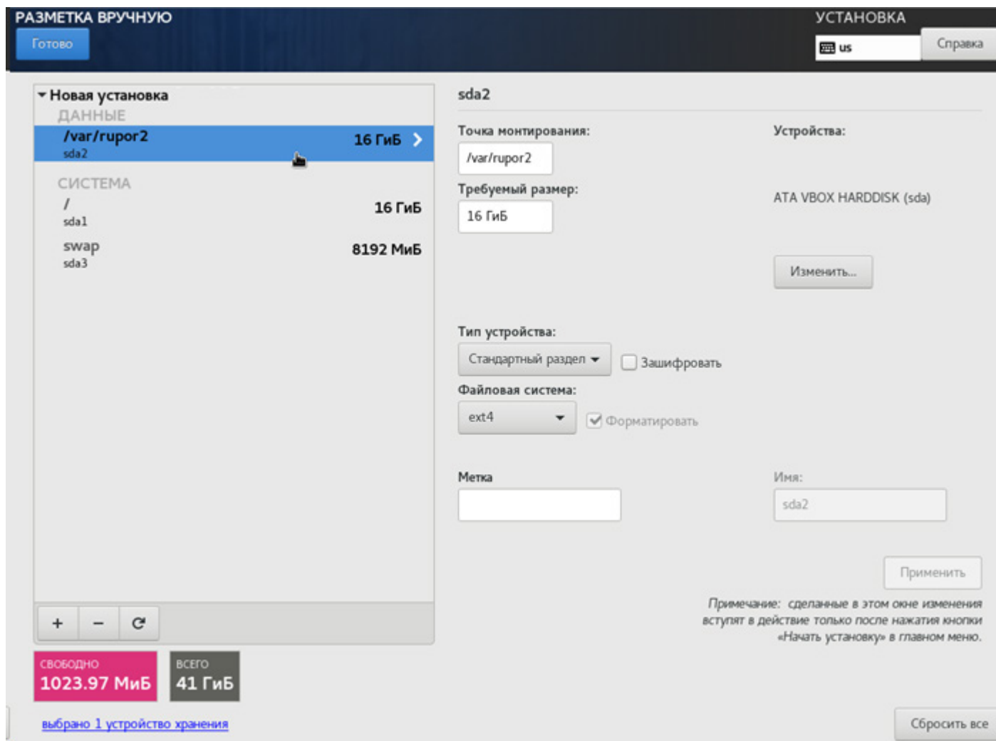
Рисунок 9 – Завершение настройки разделов
