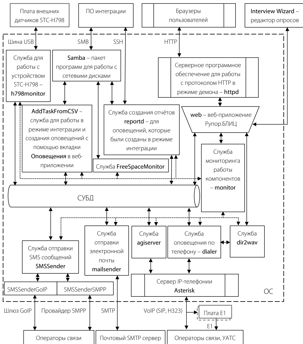
Рисунок 2 – Взаимодействие компонентов комплекса Рупор.БЛИЦ между собой и с другими системами
