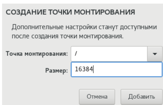
Рисунок 7 – Окно Создание точки монтирования
