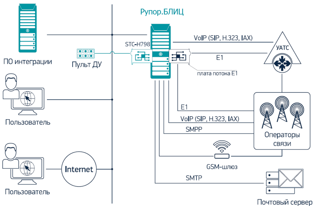
Рисунок 1 – Общая архитектура комплекса Рупор.БЛИЦ и его взаимодействие с другими системами
