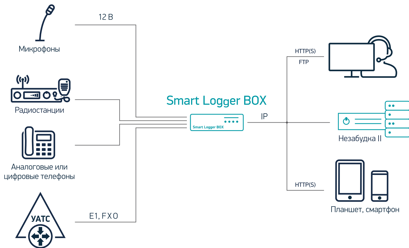
Схема развёртывания аудиосервера Smart Logger BOX
